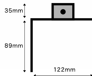
●3.5~4寸角兼用受金具
